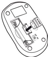
Joon. 6. Ressiiveri paigaldamine hiire korpuse sisse.
